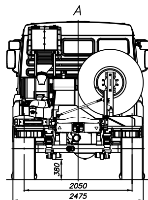
1. Размеры для справок 2.* Размеры для а/м снаряженной массы.
